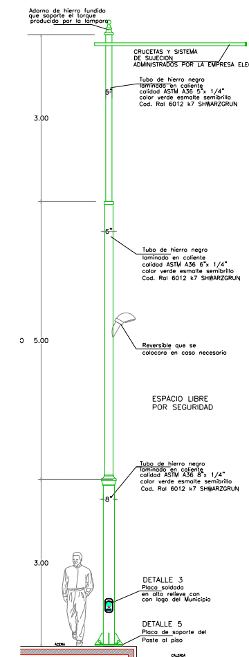
ELEVACION POSTE UNIFICADO TIPO PU-3 PU-3A CON REVERSIBLE 2 UNIDADES PU-3B SIN REVERSIBLE 2 UNIDADES ESCALA 1:20
