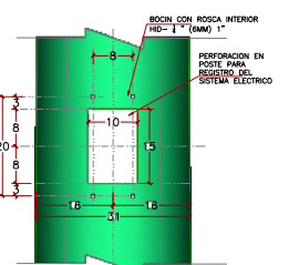
Elevación.2
