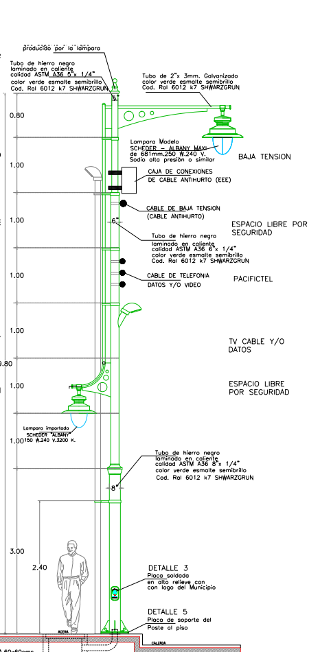
ELEVACION POSTE UNIFICADO TIPO PU-1 PU-1 20 UNIDADES ESCALA 1:20
