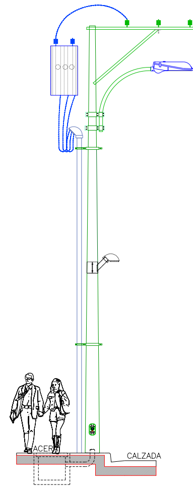
POSTE DE HORMIGON
