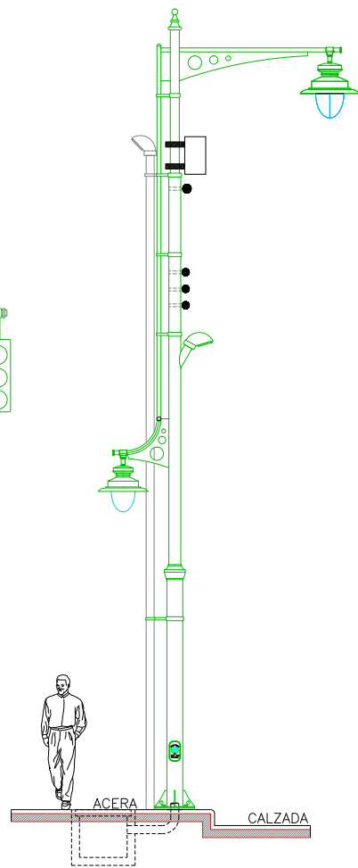
POSTE METALICO II
