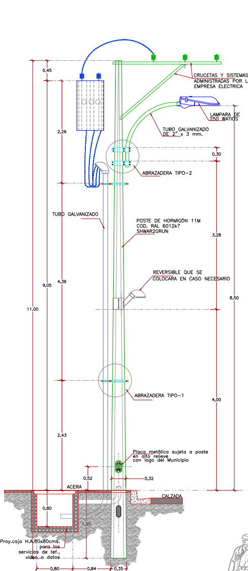
Poste Unificado DIMENSIONADO escala 1:25
