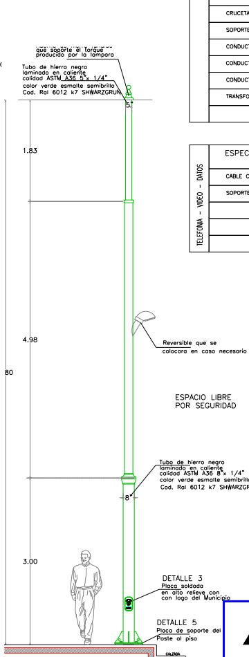
ELEVACION POSTE UNIFICADO TIPO PU-4 PU-4A CON REVERSIBLE 1 UNIDAD PU-4B SIN REVERSIBLE 4 UNIDADES ESCALA 1:20
