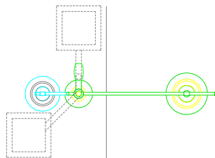
PLANTA POSTE UNIFICADO TIPO PU-1 ESCALA 1:20
