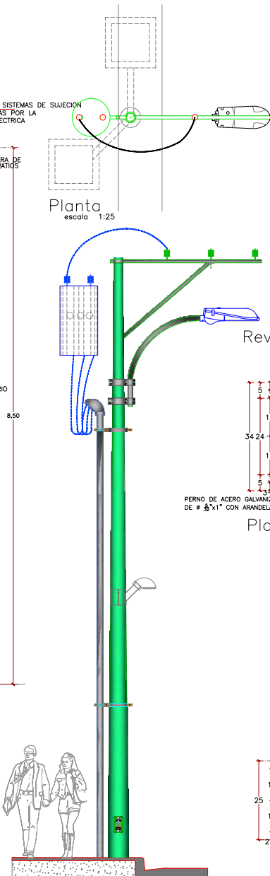
Elevación
