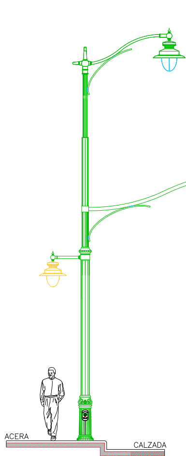
POSTE METALICO I (ORNAMENTAL)
