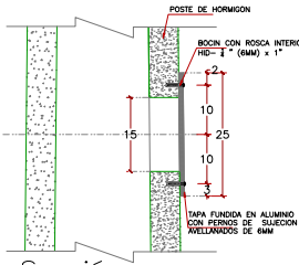
Sección
