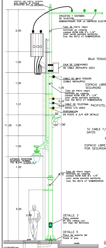
ELEVACION POSTE UNIFICADO TIPO PU-2 PU-2 15 UNIDADES ESCALA 1:20
