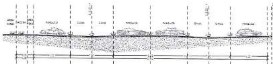
Imagen 8: Sección Típica de la Vía Corte B Elaborado por: Equipo consultor
