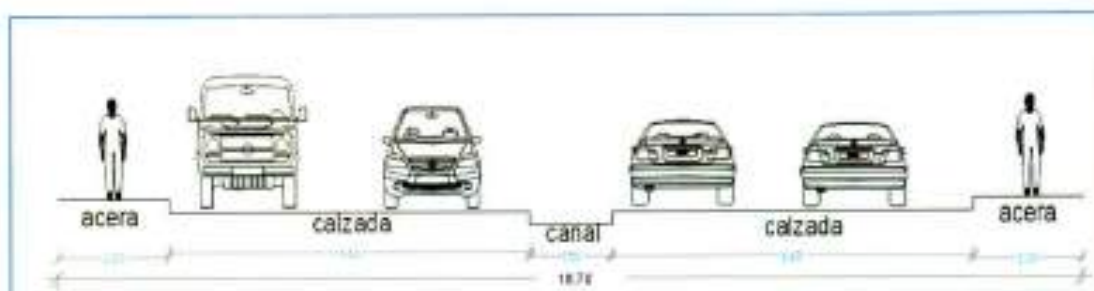
Imagen 06.- Propuesta de diseño de sección de la calle A frente al proyecto Fuente: EIV
