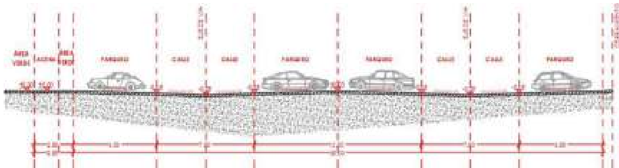
Ilustración 27. Sección Típica de la Vía Corte B. Elaborado por: Equipo consultor.
