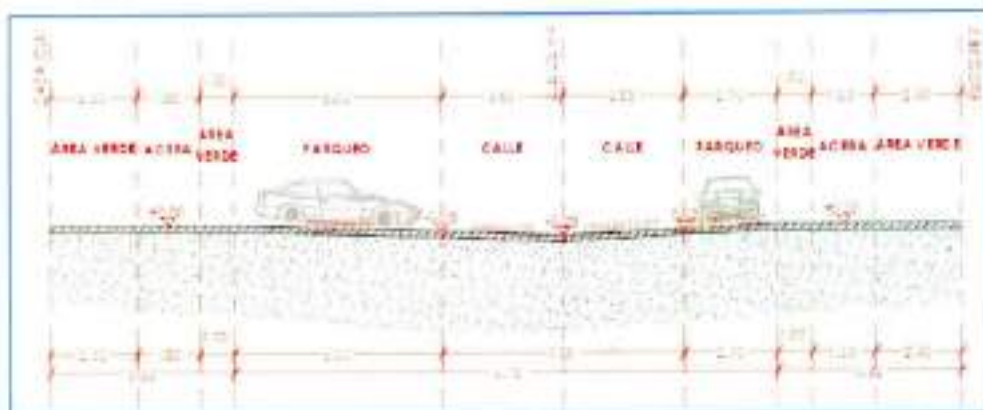
Imagen 10.- Sección de Vía Tipo C Fuente: EIV
