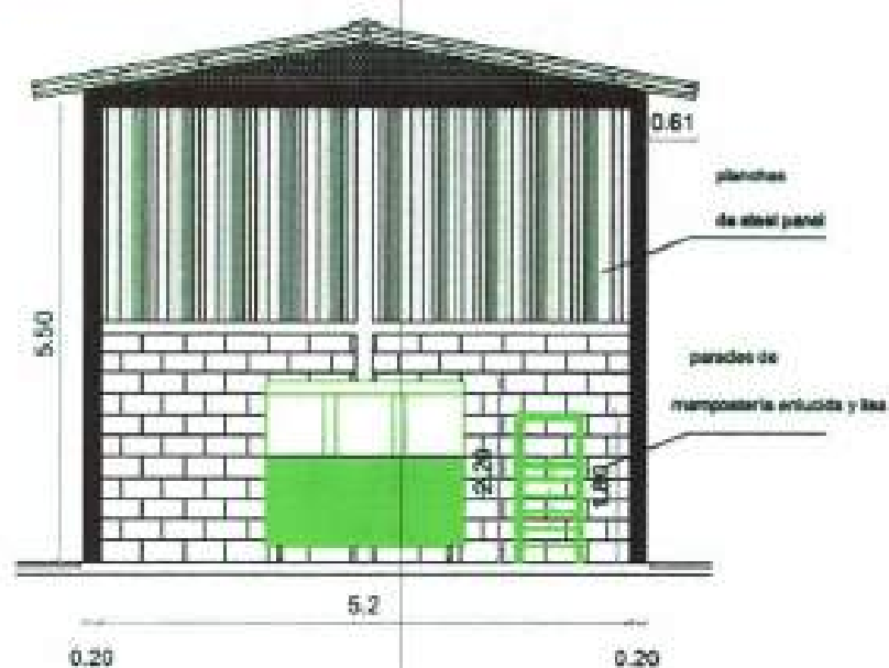
CORTE TRANSVERSAL
