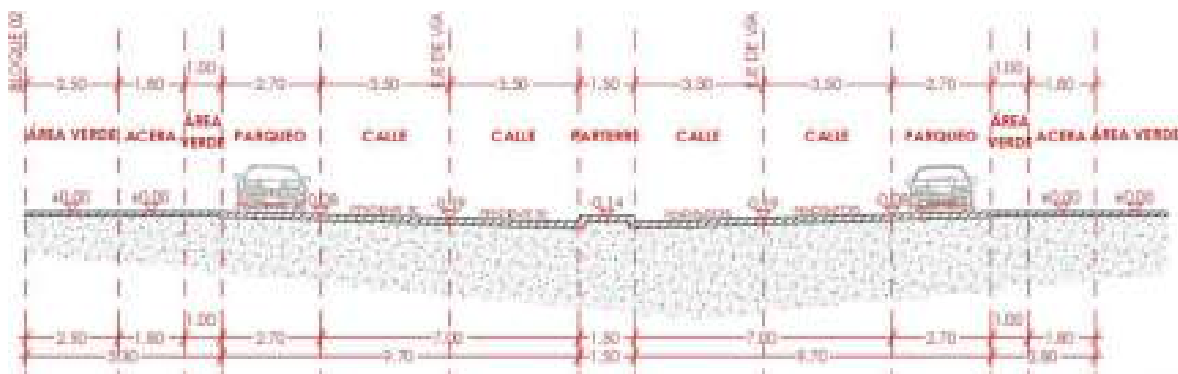
Ilustración 26: Sección Típica de la Vía Corte A, acceso y salida. Elaborado por: Equipo consultor.
