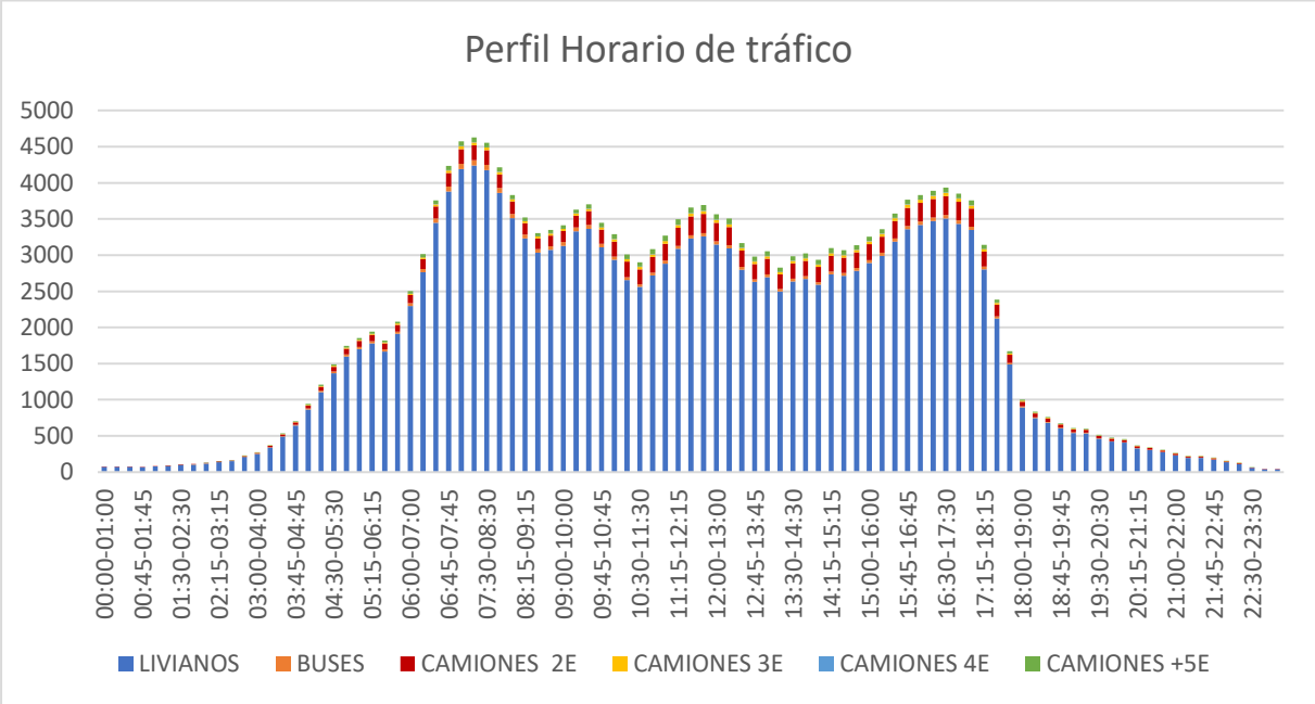
Gráfico 3: Perfil horario típico en el sentido Oeste - Este hacia Guayaquil Elaborado por: Equipo consultor
