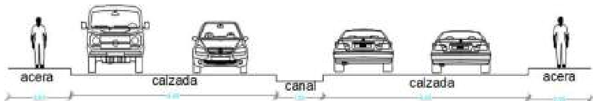
Ilustración 24: Sección de la Vía Pública de Acceso al Proyecto.
