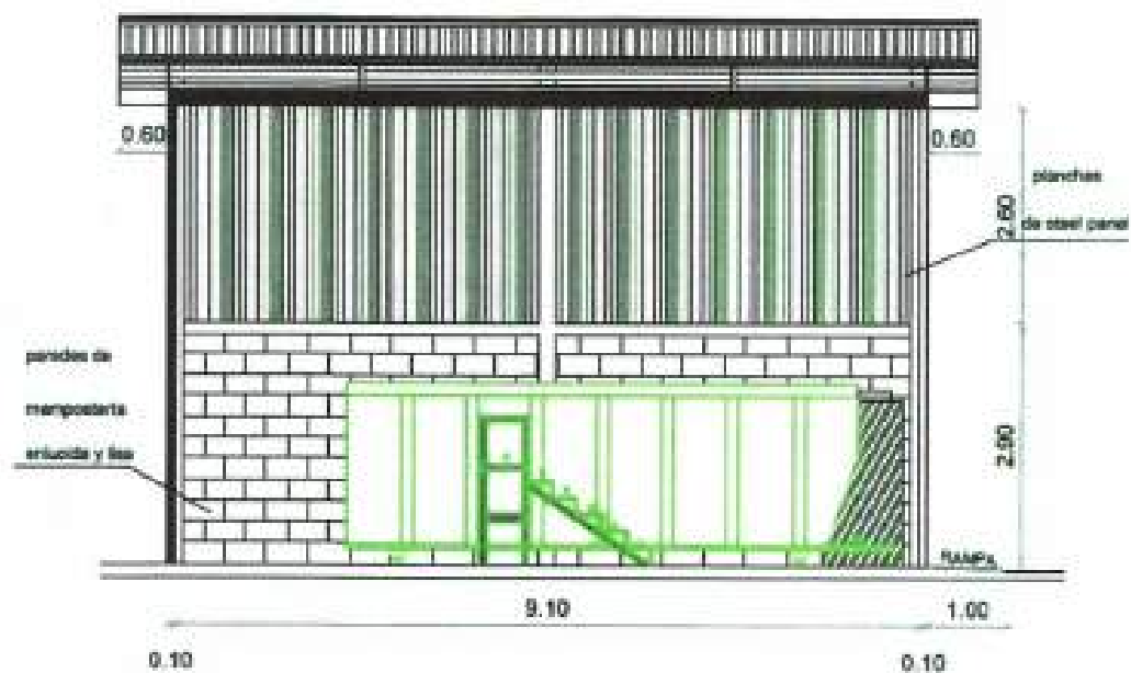
CORTE LONGITUDINAL
