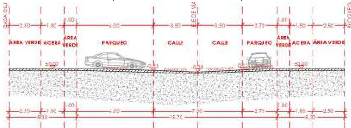
Ilustración 28: Sección Típica de la Vía Corte C. Elaborado por: Equipo consultor.
