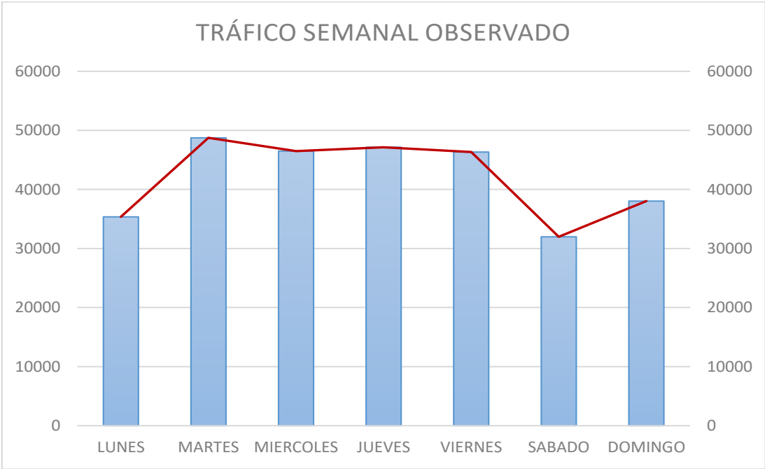
Gráfico 2: Comportamiento del tráfico por días en la semana hacia Guayaquil Elaborado por: Equipo consultor
