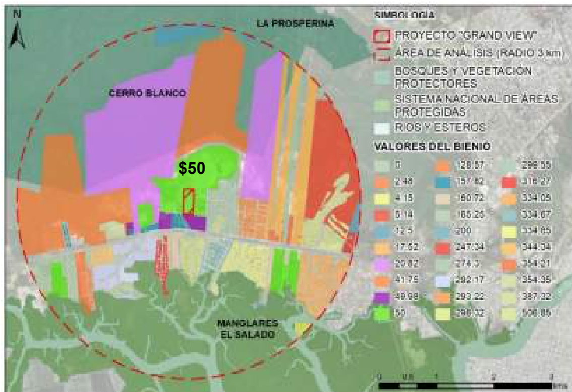
Ilustración 2: Estructura Predial del área de diagnóstico del Plan Parcial Grand View.
