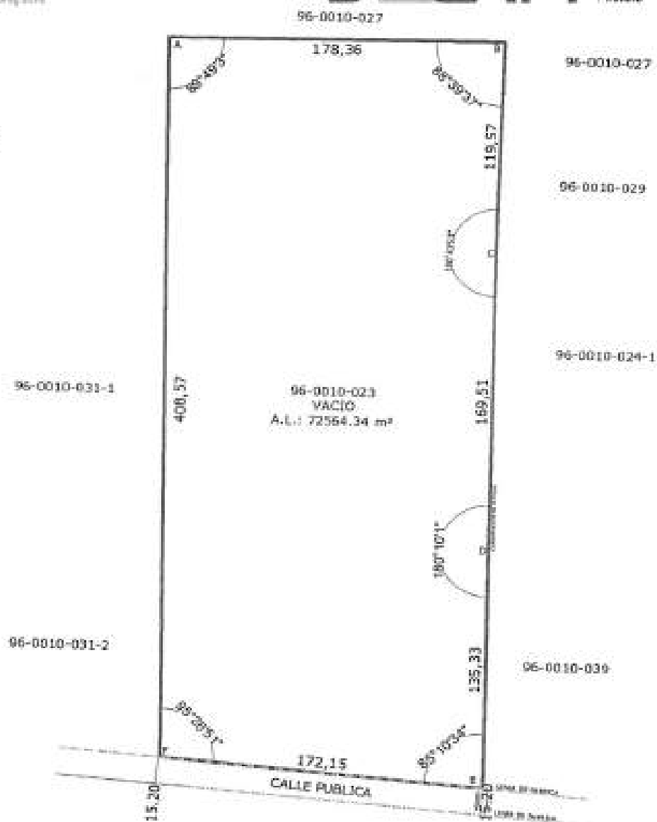
Figura 1. Levantamiento topográfico realizado por el departamento de topografía.
