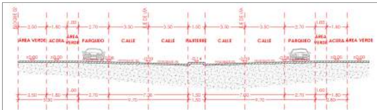
Imagen 7: Sección Típica de la Vía Corte A, acceso y salida Elaborado por: Equipo consultor
