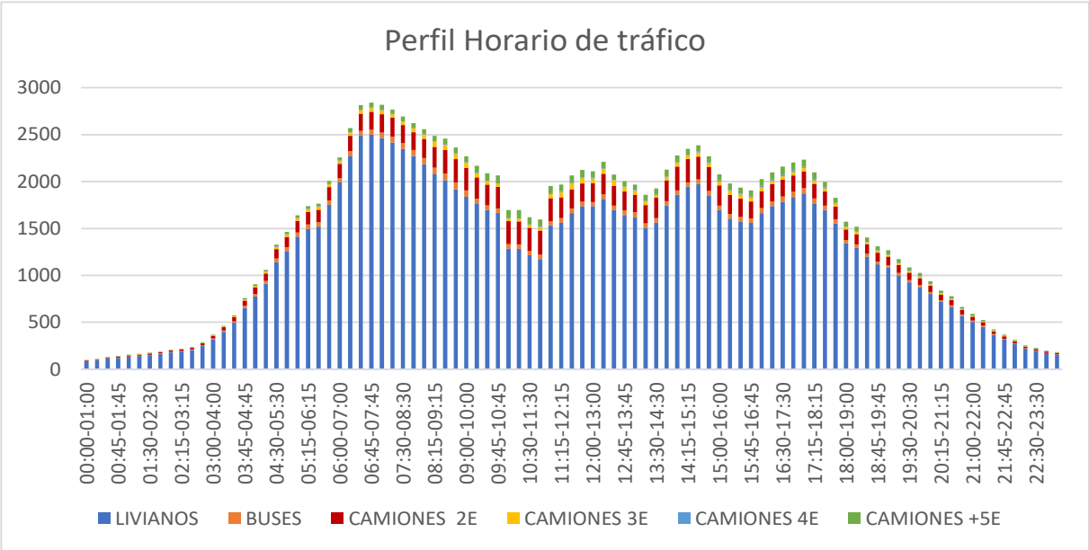
Gráfico 6: Perfil horario típico en el sentido Este - Oeste, hacia Chongón Elaborado por: Equipo consultor
