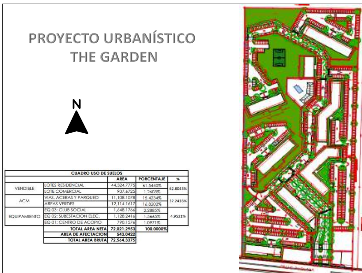
Imagen 3: Implantación arquitectónica General del Proyecto
