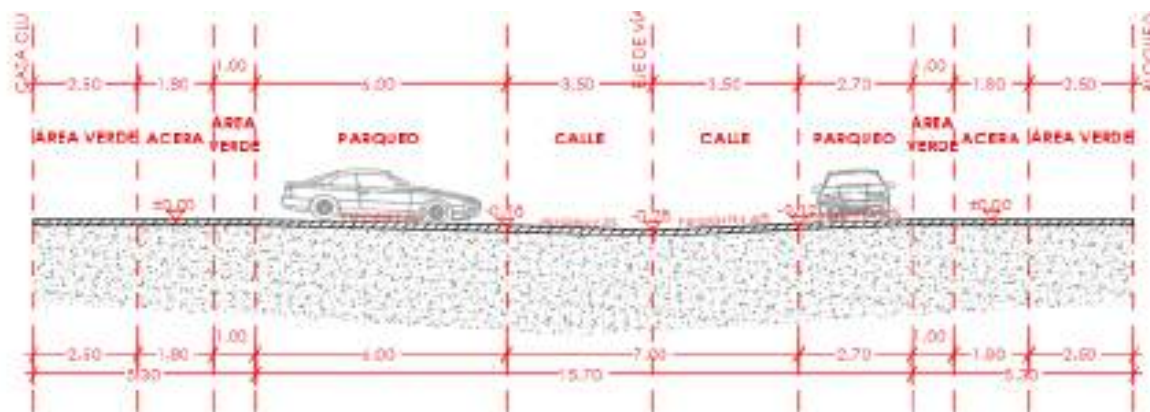
Imagen 9: Sección Típica de la Vía Corte C Elaborado por: Equipo consultor
