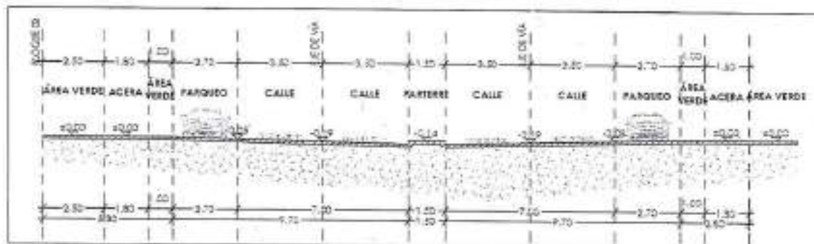
Imagen 7: Sección Típica de la Vía Corte A, acceso y salida Elaborado por: Equipo consultor
