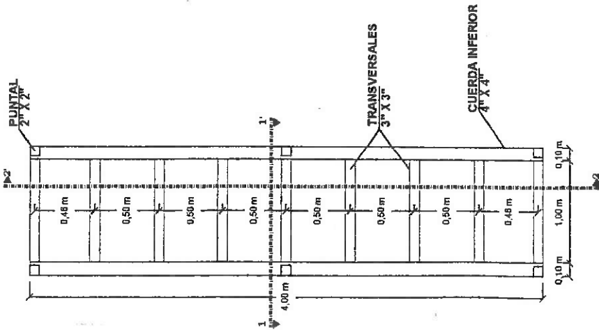
PLANTA
