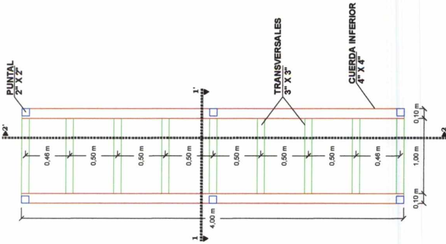
PLANTA
